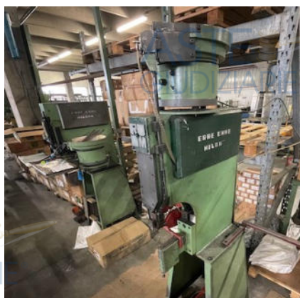
Id 23 – Rivettatrice
