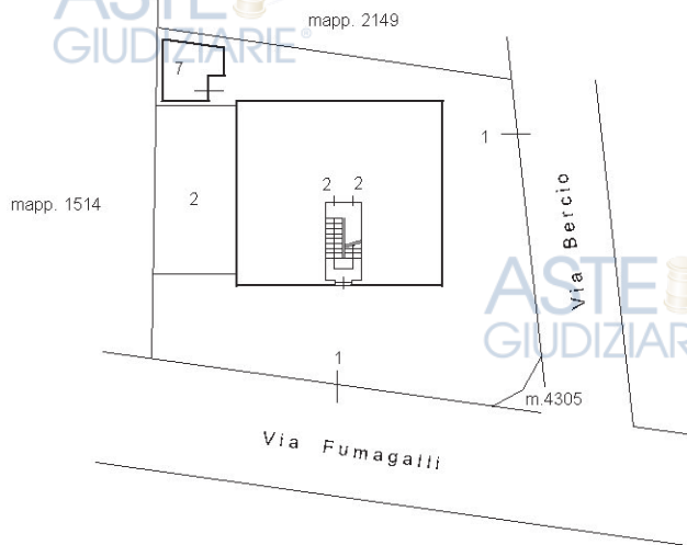
Piano Terra (Rialzato)
