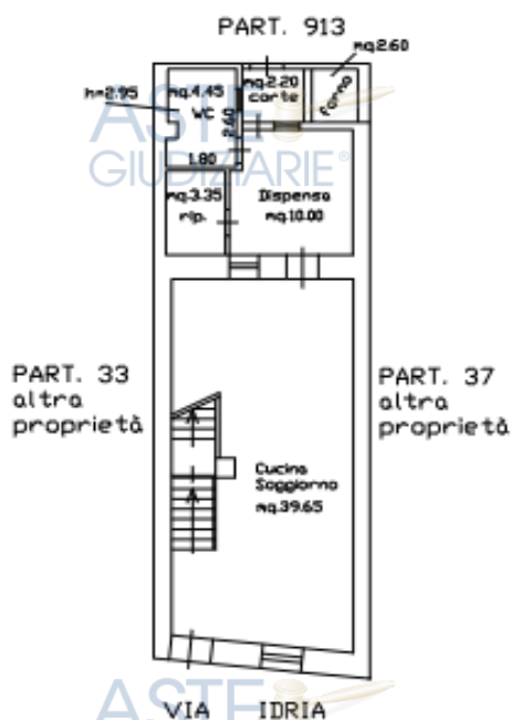
PIANO TERRA STATO ESISTENTE H=3.40
