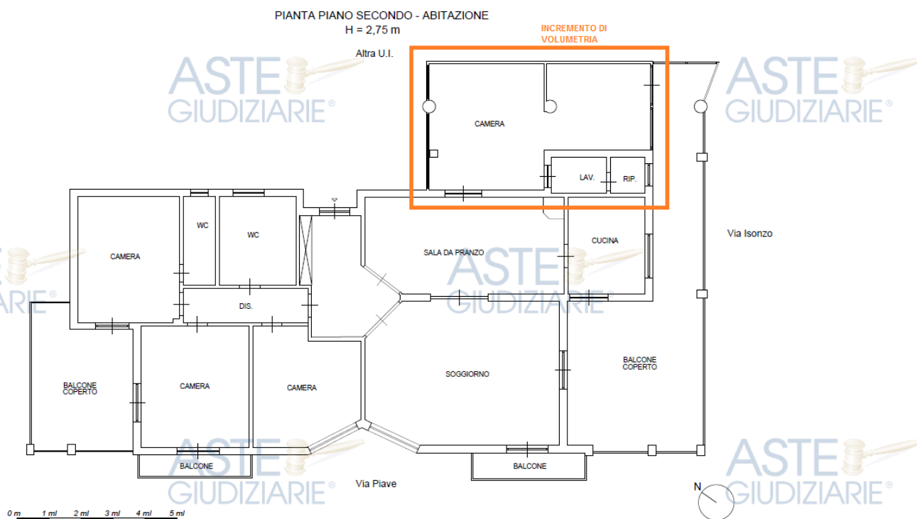
FIGURA 1. Planimetria stato dei luoghi del bene n.1 con individuazione dell'incremento di volumetria
