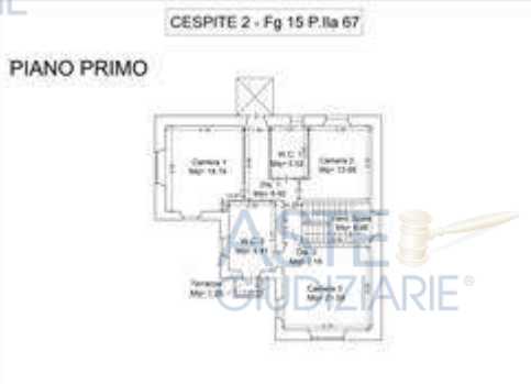
Planimetria piano primo con misure rilevate
