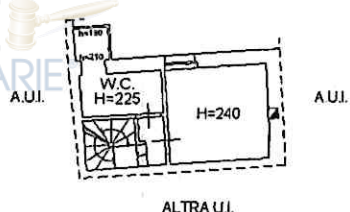
PIANTA PIANO TERZO
