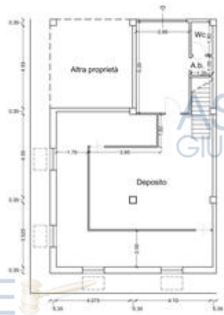
PIANTA PIANO INTERRATO | h: 3.50 mt
