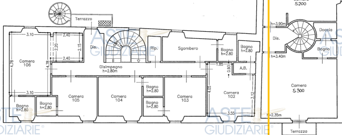
PIANTA PIANO PRIMO H = 2.90 m
