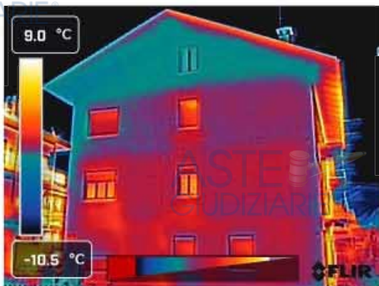
Foto 19 – Termografia ovest edificio
