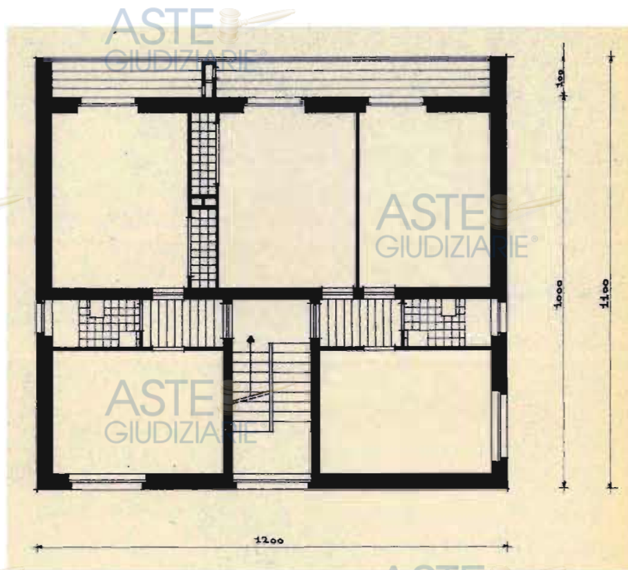
Estratto grafico del progetto autorizzato - Piano "tipo"
