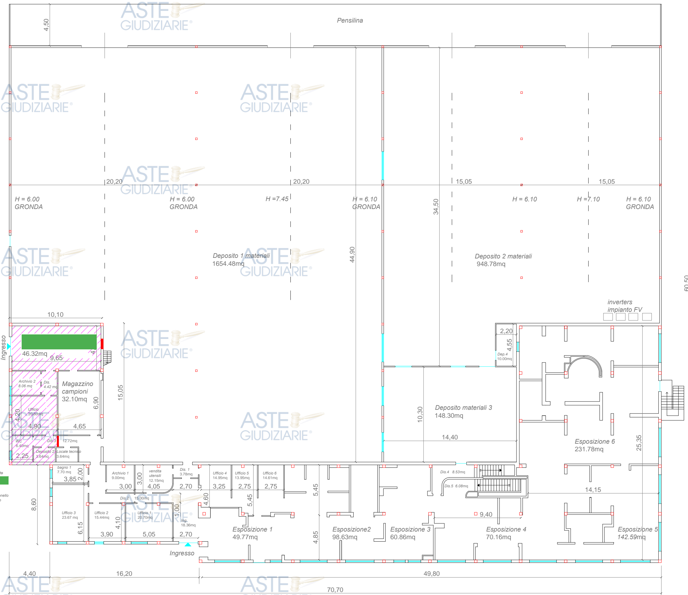
Pianta Piano terra fuori scala
