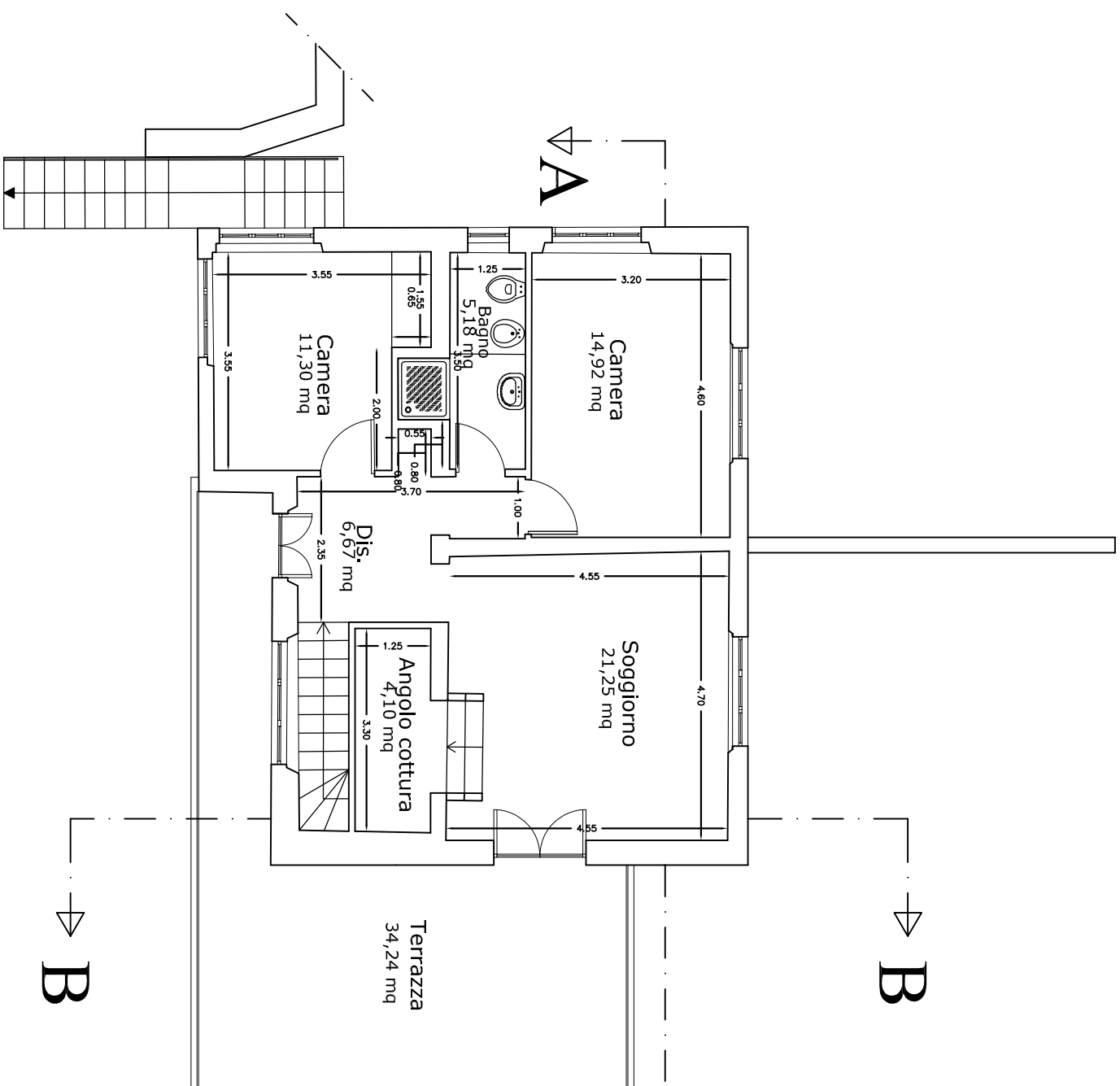
PIANO PRIMO
