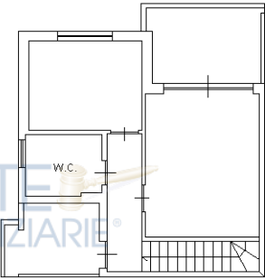
PIANO PRIMO H= 2.70
