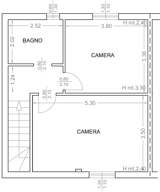
Piano Primo
