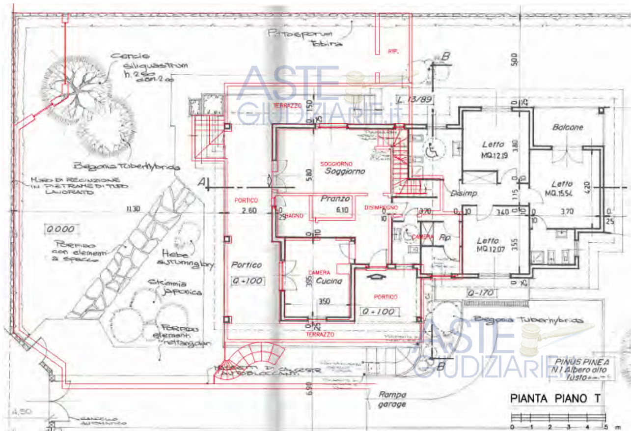
Sovrapposizione della restituzione del rilievo eseguito al grafico allegato alla concessione n. 889/C/2001
