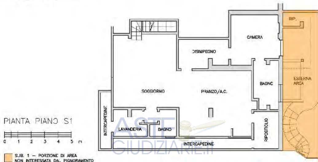
La restituzione del rilievo effettuato (non in scala)
