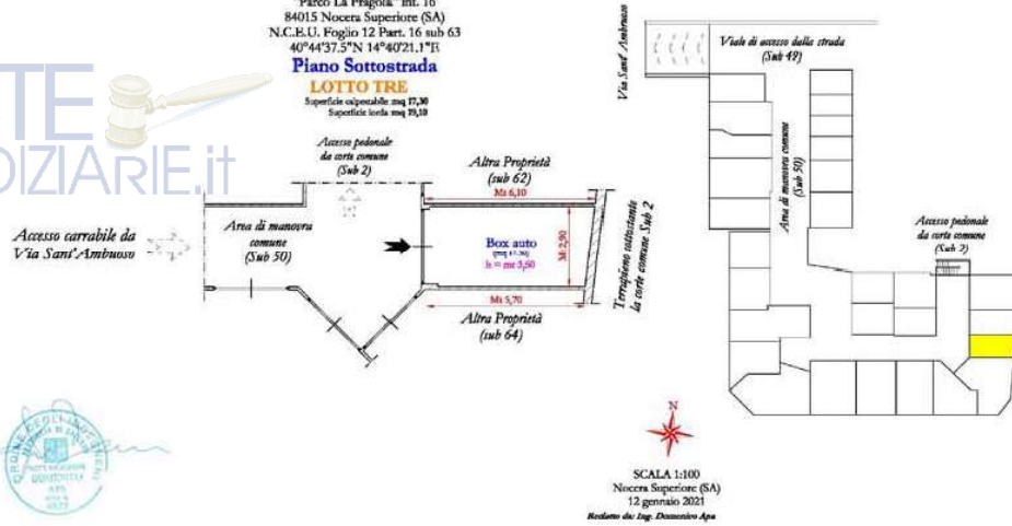
Planimetria Posto Auto
